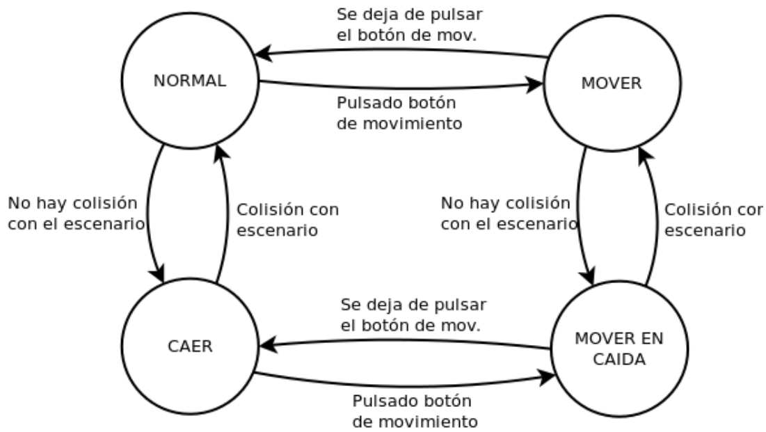
Figura 3: Sencillo autómata de ejemplo para el comportamiento de un actor
